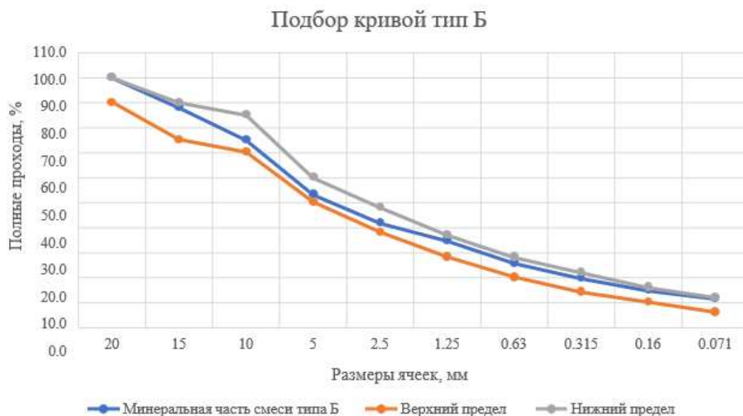
Рисунок 1 - Гранулометрический состав выбранного асфальтобетона тип Б
