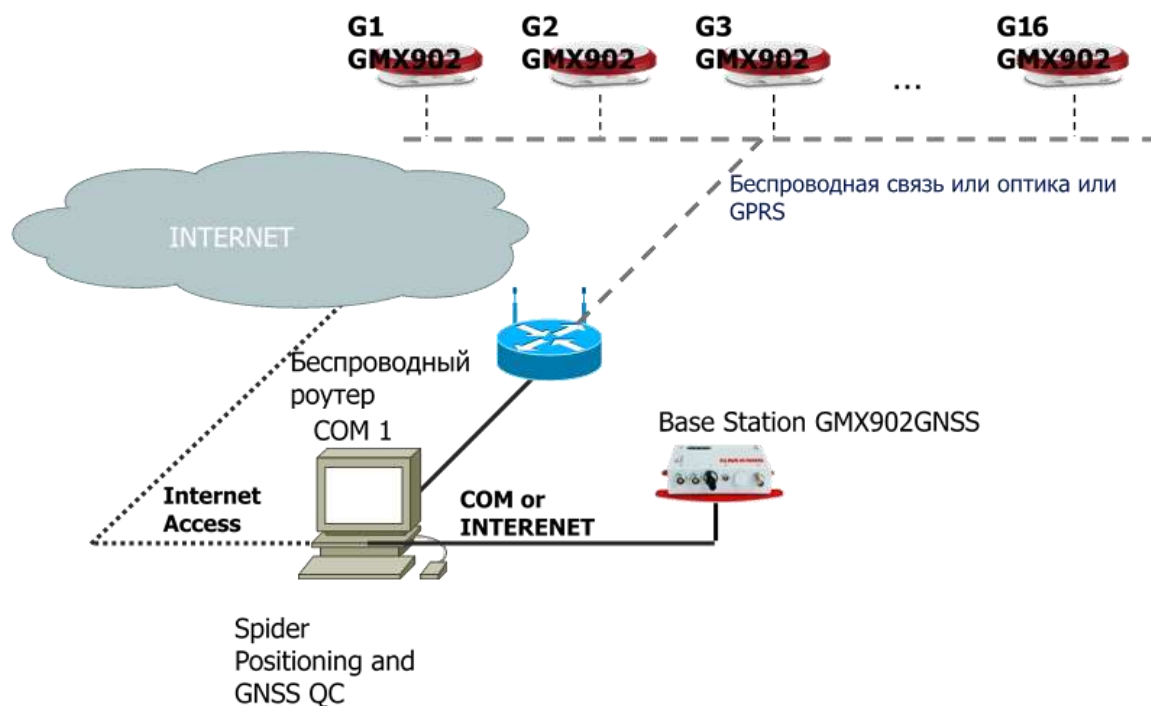
Рис. 4. Принцип работы ГНСС оборудования автоматизированной системы деформационного мониторинга на мосту Александра Невского
