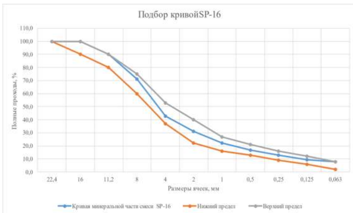
Рисунок 2 - Гранулометрический состав подобранного асфальтобетона тип SP-16
